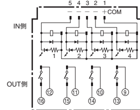
端子配置/内部接线图 (顶视图)
